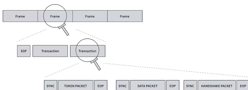
12. ábra. USB frame[19]
