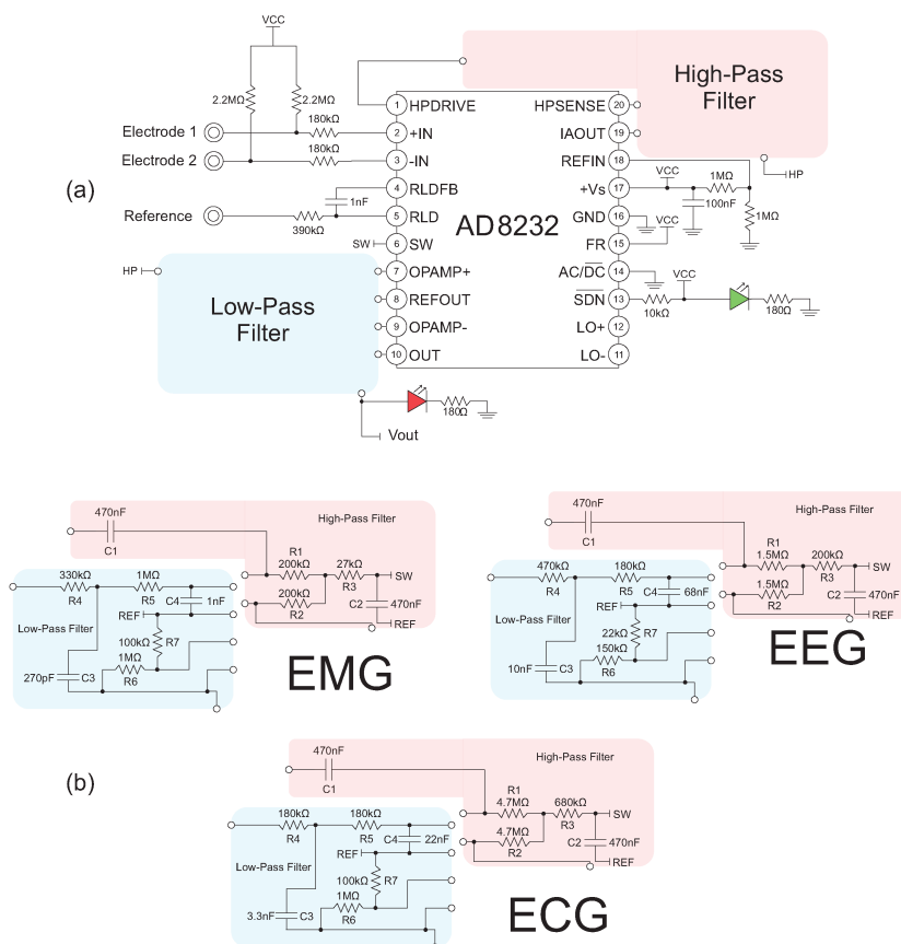
7. ábra. A cikkben leírt megfelelő EMG konfigurációt követtük[17]
